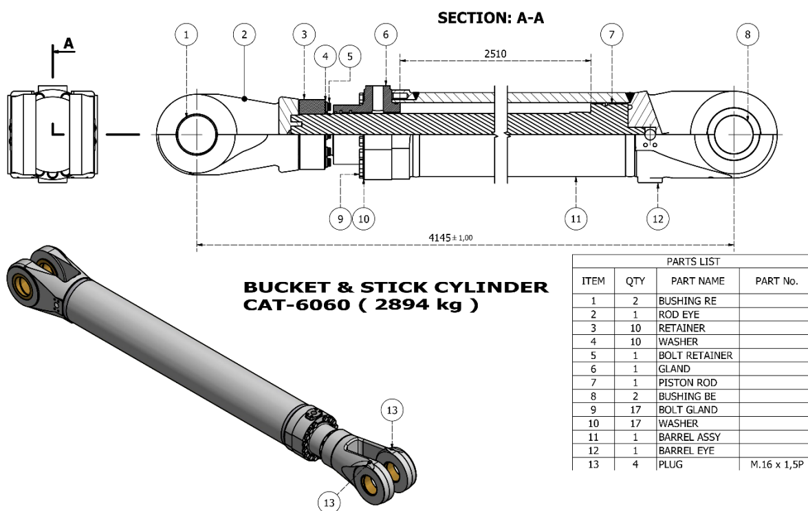
Зураг 2 Гидравлик цилиндр
