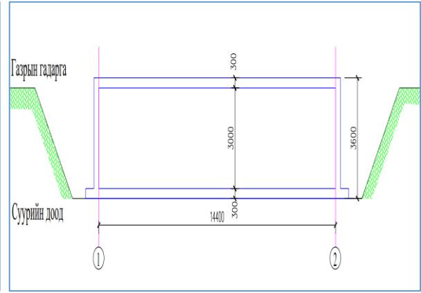
Зураг 6.7, 6.8. Бетонон хучилттай MNS5924:2005 стандартын шаардлага хангасан нүхэн жорлон, далд ажлын зураг
