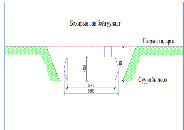
Зураг 6.9, 6.10. Бохир усны септик танк, далд ажлын зураг
