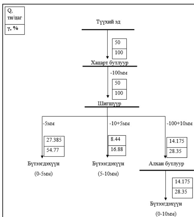
Зураг 4. Нүүрс бутлан ангилах үйлдвэрийн технологийн шат дамжлагын схем
