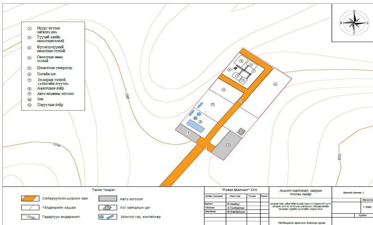
Зураг 3. Үйлдвэрийн ерөнхий төлөвлөлтийн зураг
