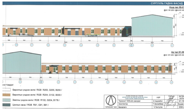
Зураг 6. Сургуулийн гадаад байгуулалт
