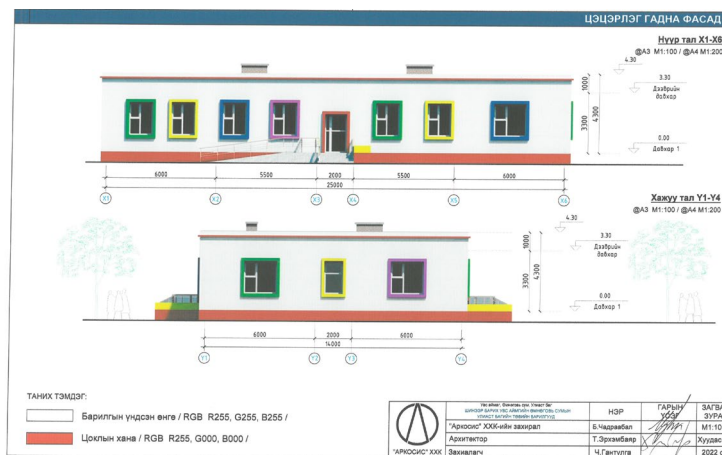
Зураг 4. Цэцэрлэгийн зохион байгуулалт
