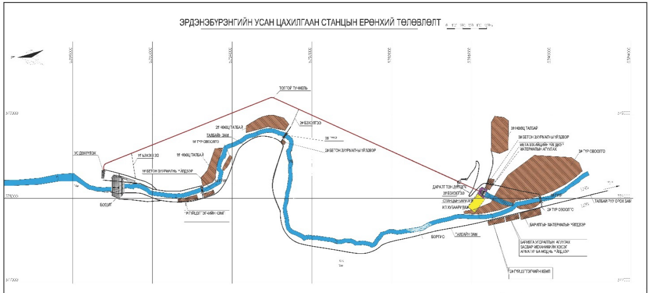
Зураг 2. Ерөнхий төлөвлөгөө
