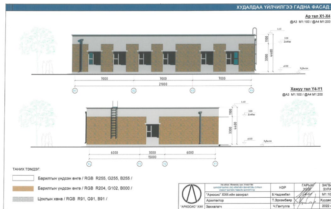
Зураг 7. Үйлчилгээний төвийн зохион байгуулалт
