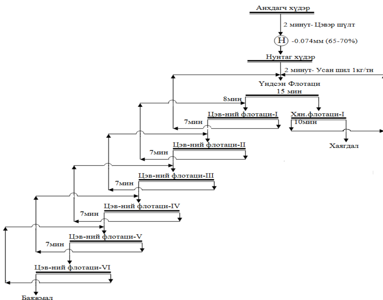
Схем №. 1 Жонш баяжуулах технологийн схем
