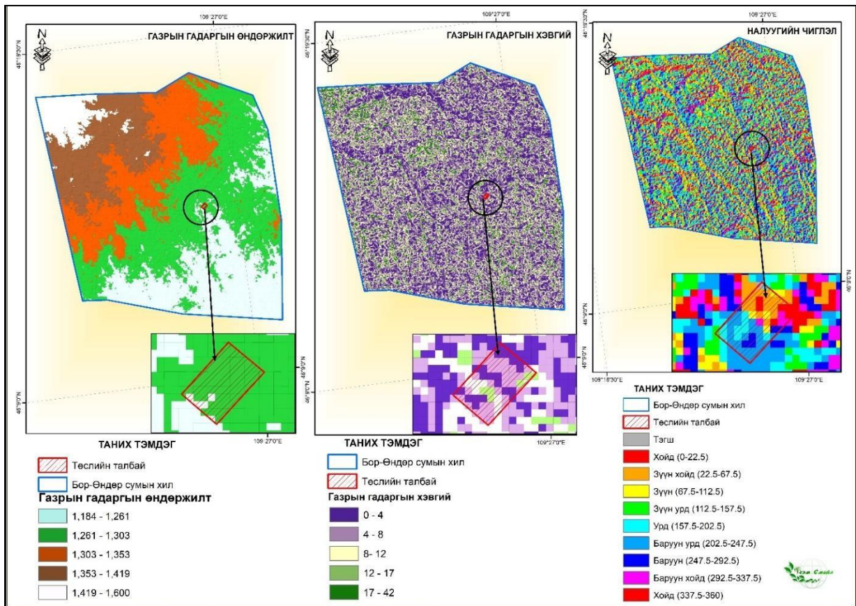
Зураг №. 5 Төсөл хэрэгжих талбайн рельеф
