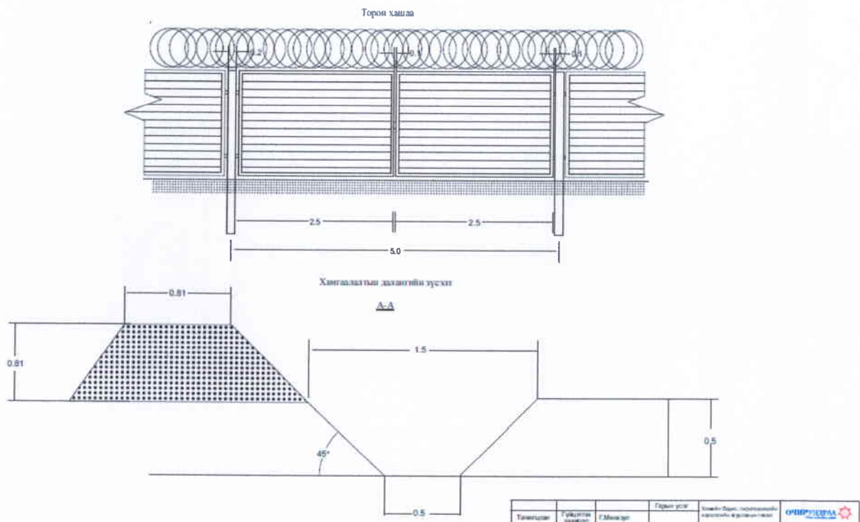
Зураг 4. Азуулахын хашаа болон үерийн уснаас хамгаалах сувгийн зураг
