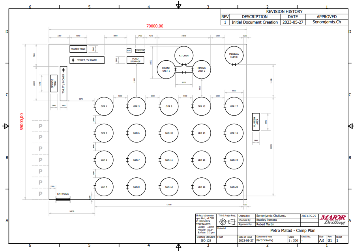
Зураг 11. Кемпийн төлөвлөлт
