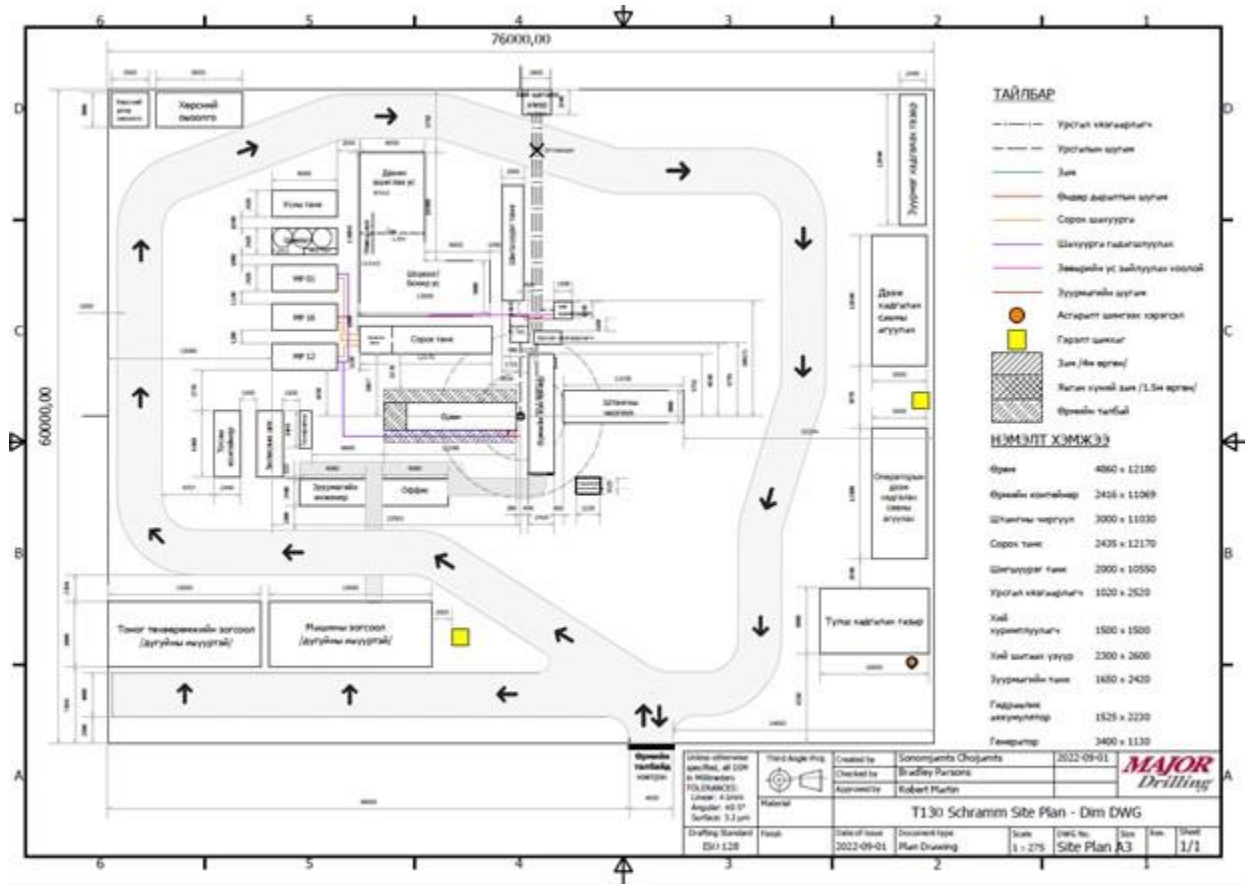
Зураг 5. Өрөмдлөгийн талбайн ерөнхий төлөвлөлт
