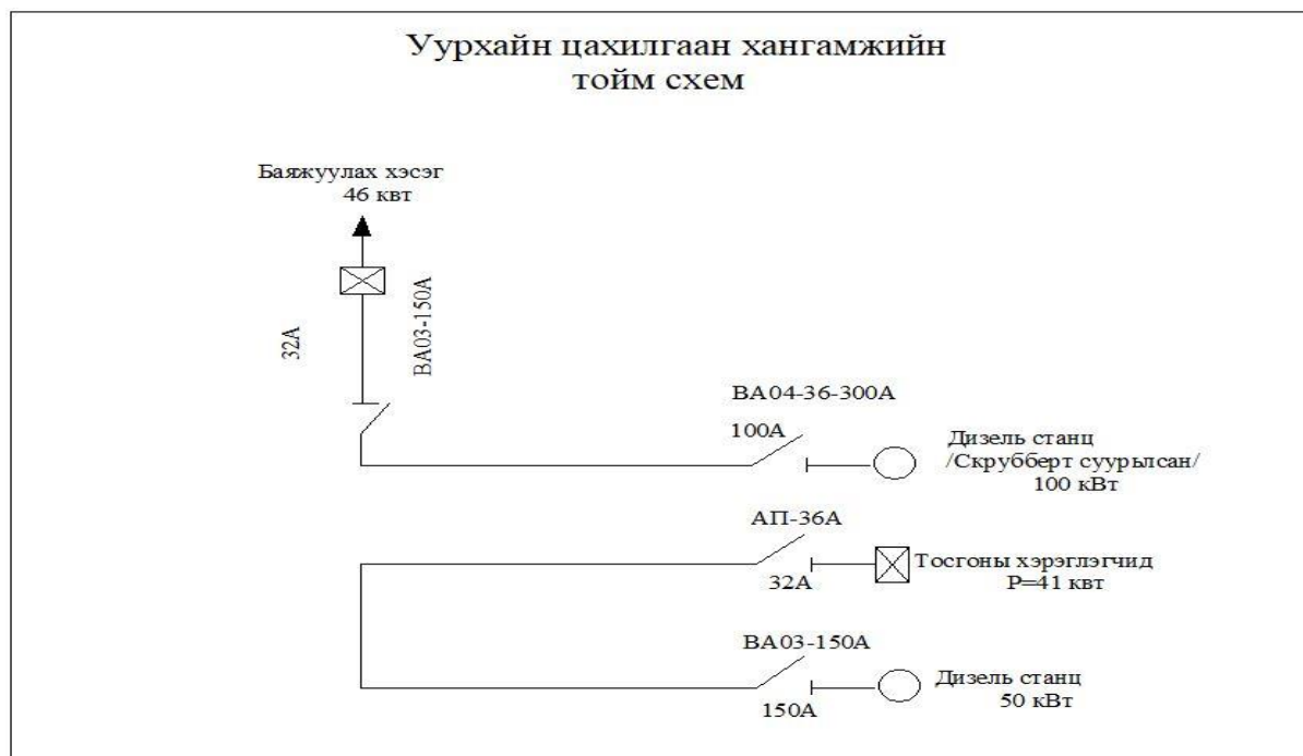
Зураг 4. Уурхайн цахилгаан хангамжийн схем
