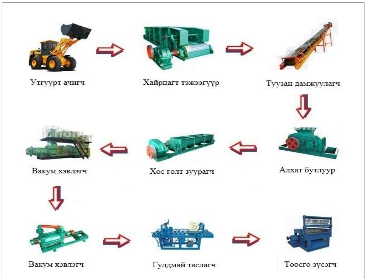
Зураг 2. Тоосго үйлдвэрлэлийн тоног төхөөрөмжийн дамжлага схем
