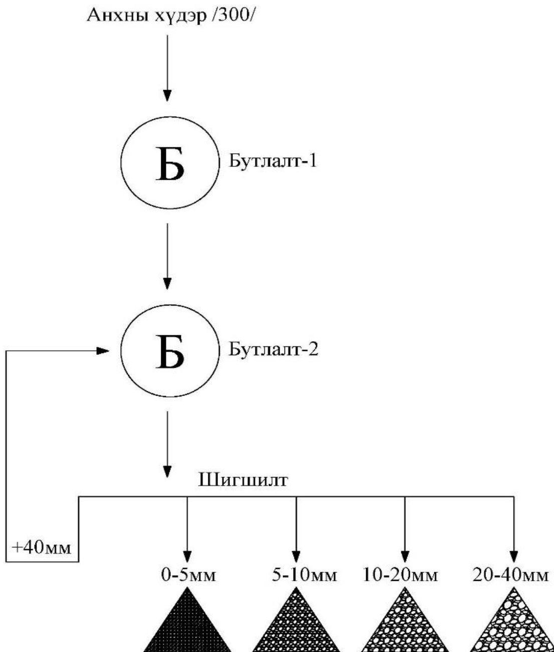
Зураг- 3. Бутлах үйлдвэрийн тоног төхөөрөмжийн технологийн схем
