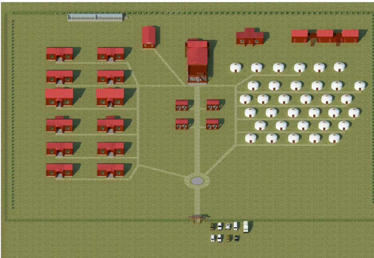
„Говь-Эрдэнэ“ баазын ерөнхий дотоод зохион байгуулалт
