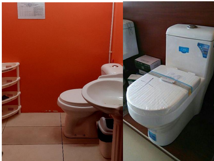
Зураг 3. Ариун цэврийн өрөөний бочкинд усны зарцуулалтыг их болон бага хувилбараар сонгох хос даралтат товчлуур суурилуулсан
