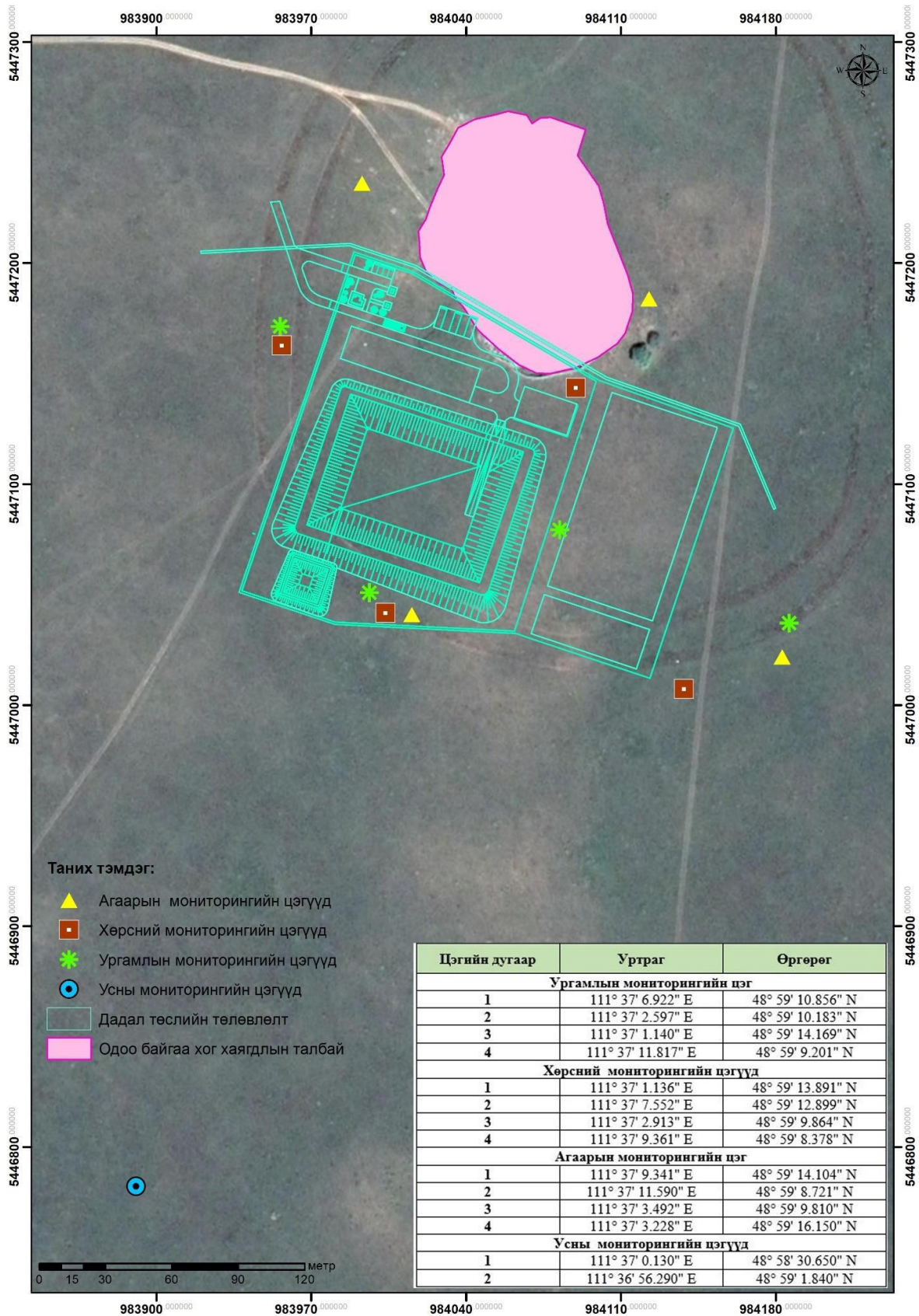
Зураг 9. Орчны хяналт шинжилгээний хөтөлбөрийн цэгүүдийн байршил
