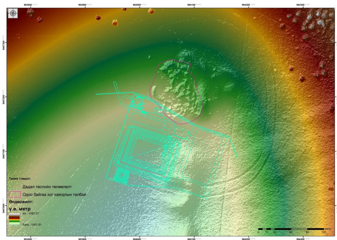
Зураг 7. Төслийн талбай орчмын өндрийн тоон загвар
