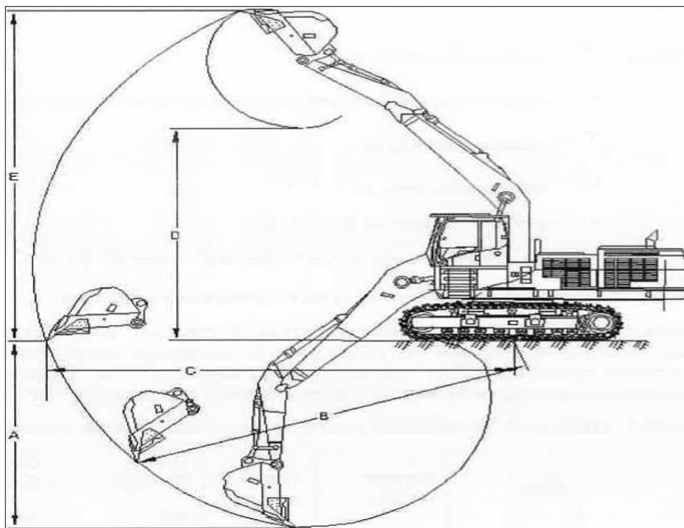
Зураг 3. CAT-325D маркийн урвуу утгуурт экскаваторын схем зураг
