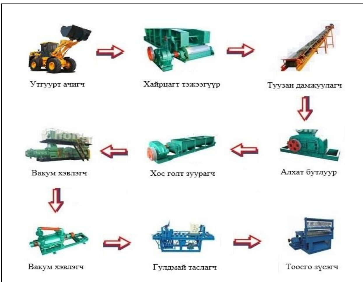
Зураг 1.3. Тоосго үйлдвэрлэлийн тоног төхөөрөмжийн дамжлага схем
