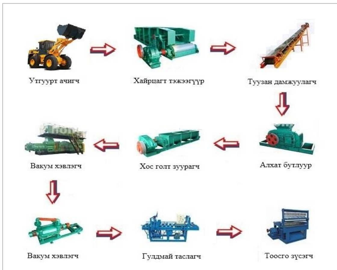
Зураг 2. Тоосго үйлдвэрлэлийн тоног төхөөрөмжийн дамжлага схем
